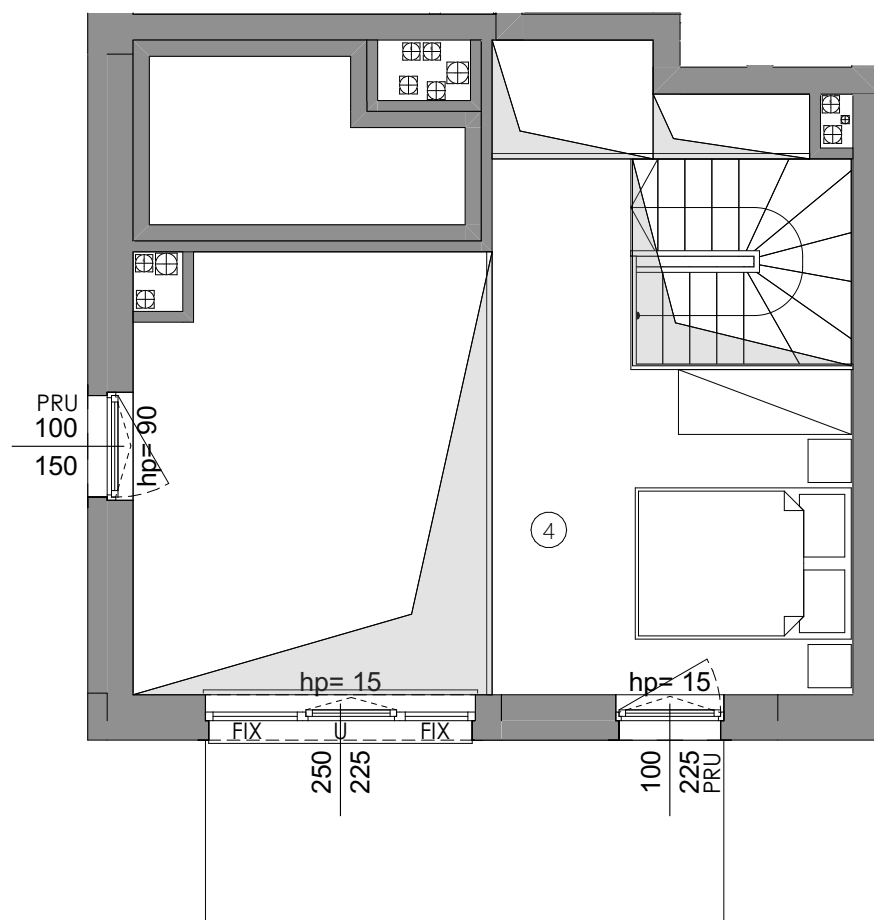
POZIOM ANTRESOLI
