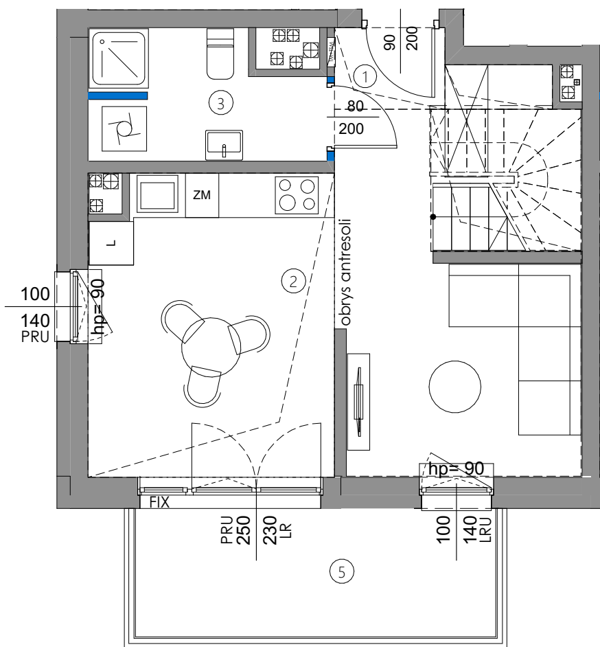
POZIOM DOLNY
