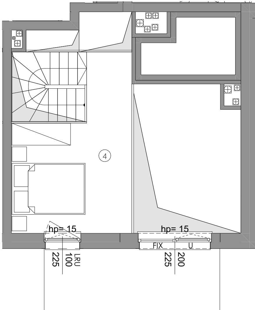
POZIOM ANTRESOLI
