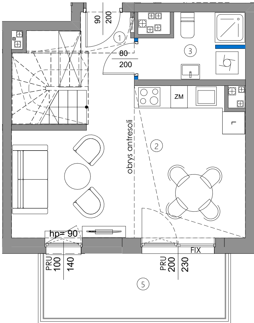
POZIOM DOLNY
