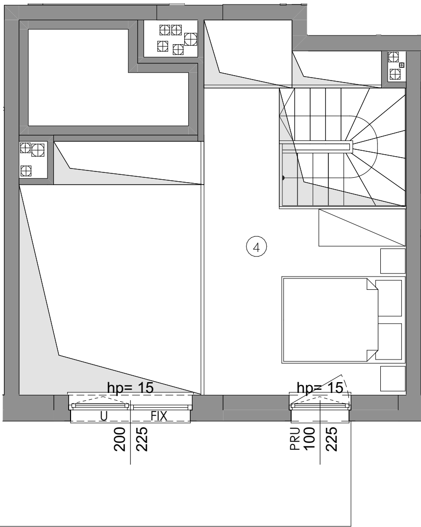
POZIOM ANTRESOLI
