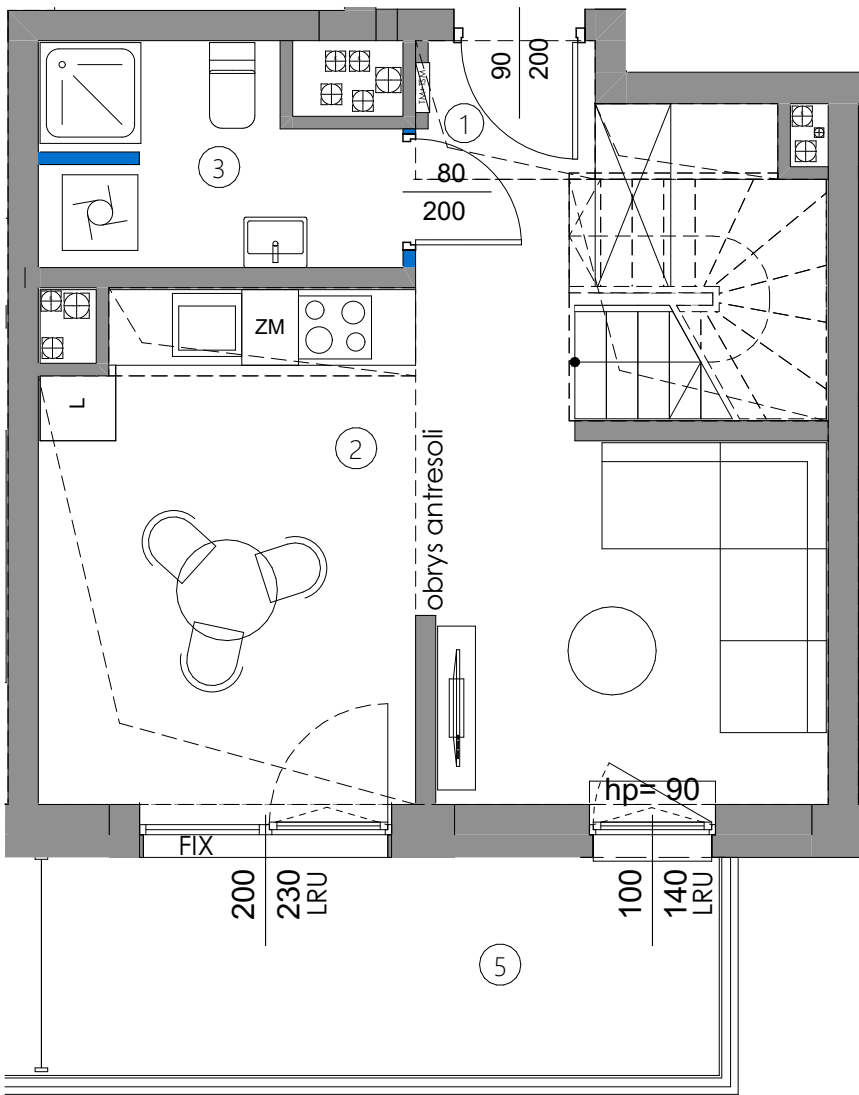
POZIOM DOLNY
