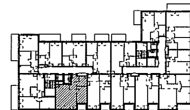
Rzut piętra 5 Kondygnacja +6
